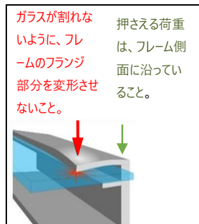
図 1a: クランプで押さえる荷重の位置
